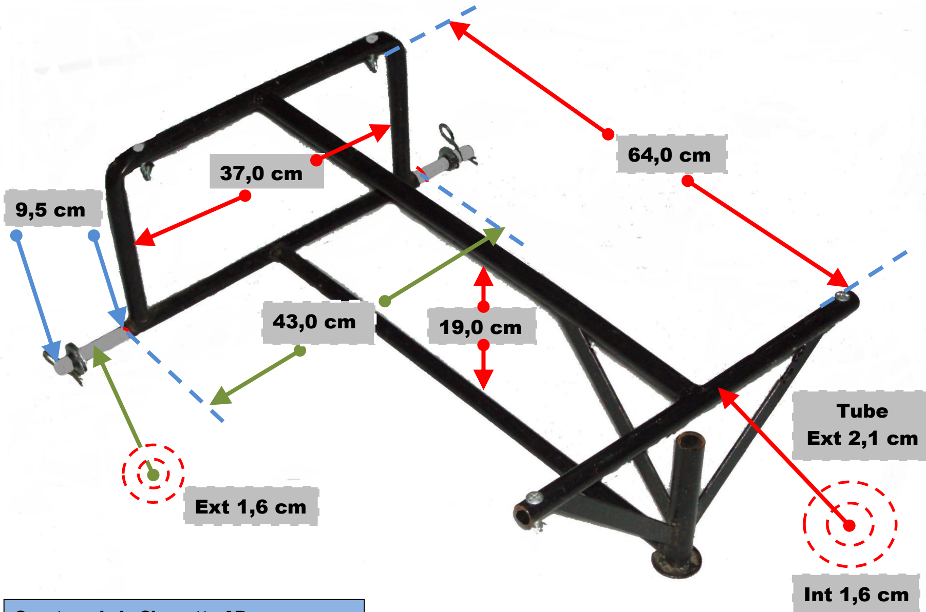
Ossature de la Charrette-AR COPYRIGHT © CLUB-ST-AGATHON-EAC Mise à jour G.A. Janvier 2012
